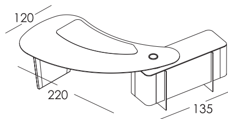
MÓDULO GIRATORIO desk: Swivel unit ADAPTABLE AL ESPACIO Adjustable to space
