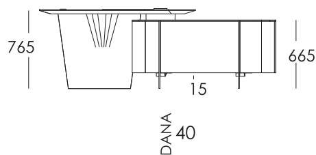
Mesa oficina con forma Shaped office desk Tapa / Top 220x120 módulo / Swivel unit 135x45xA64 Ref 191.DE220
