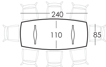
Mesa de 240 Table 240w Ref 191.AX240 Puntos 1372
