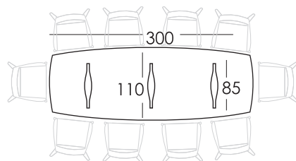
Mesa de 300 Table W300cm Ref 191.AX300
